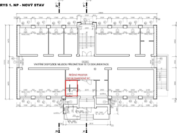
PŮDORYS 1. NP - NOVÝ STAV
